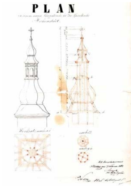
Plány na bání věže 1862. Okresní archiv Šumperk, fond farnosti Zábřeh.
